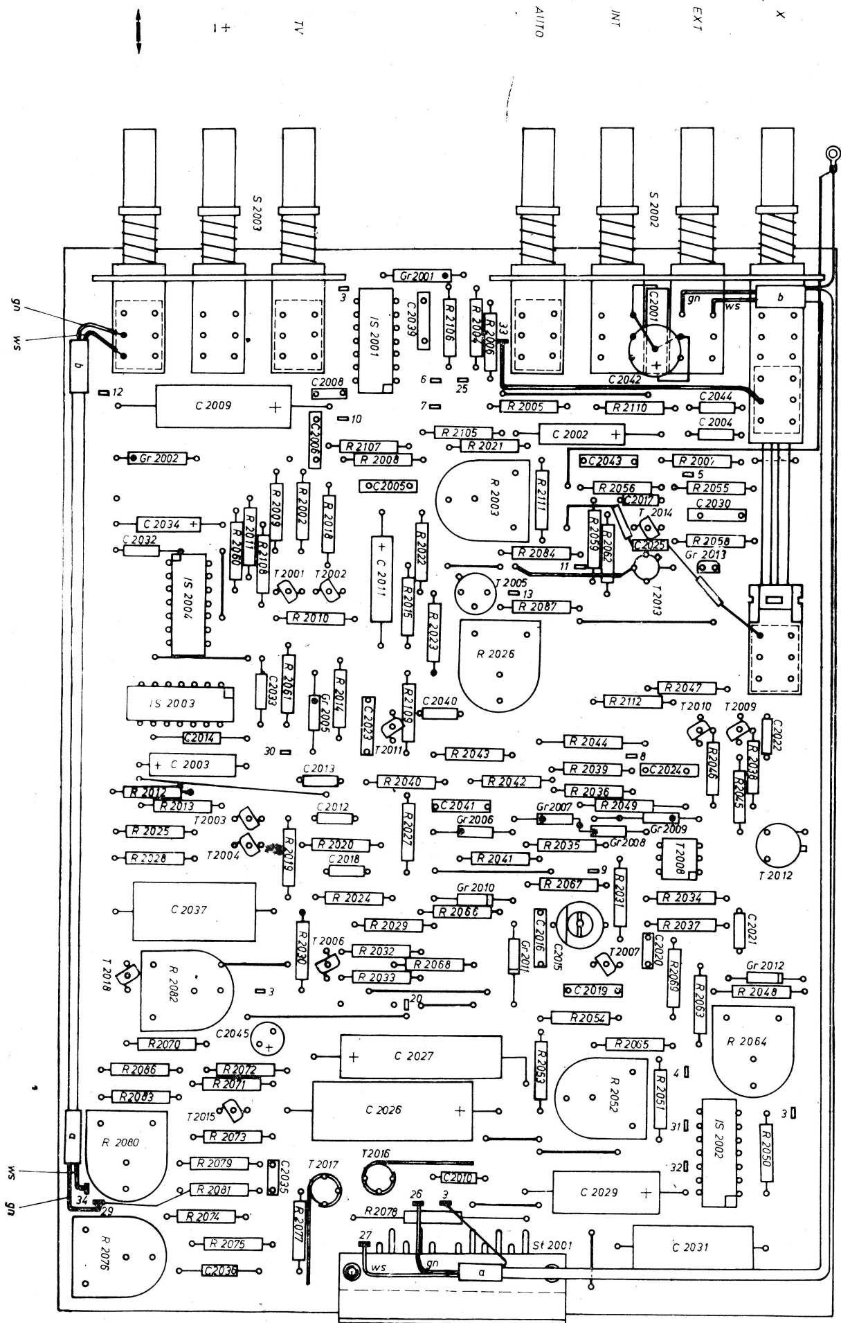
Leiterplatte X-Kassette
