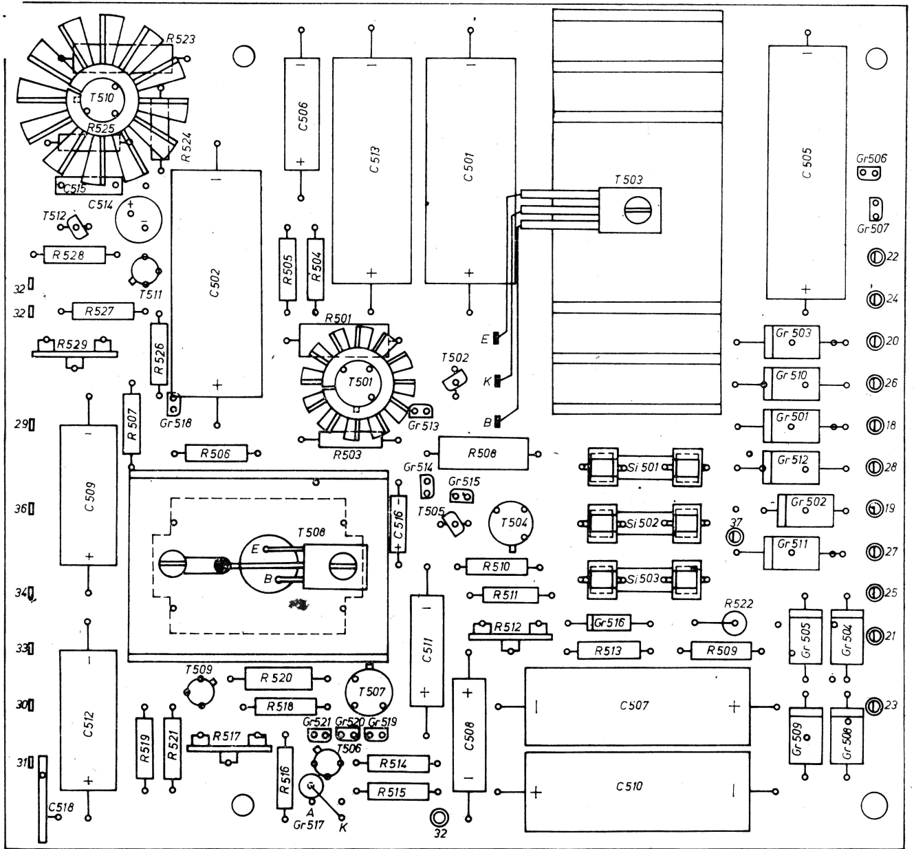
Leiterplatte Netzteil
