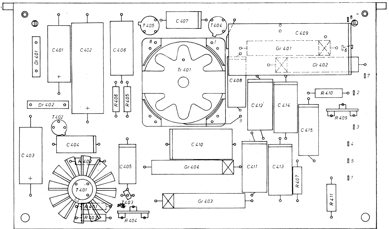
Leiterplatte Transverter
