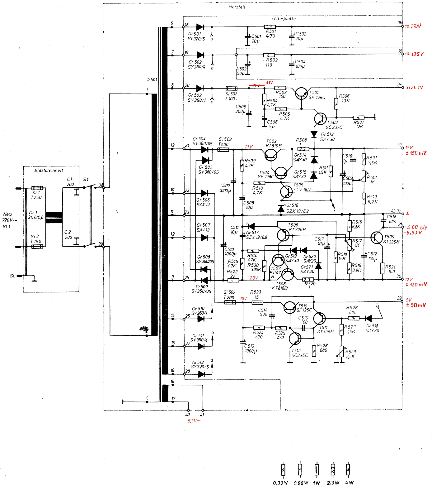
Stromlaufplan Netzteil
