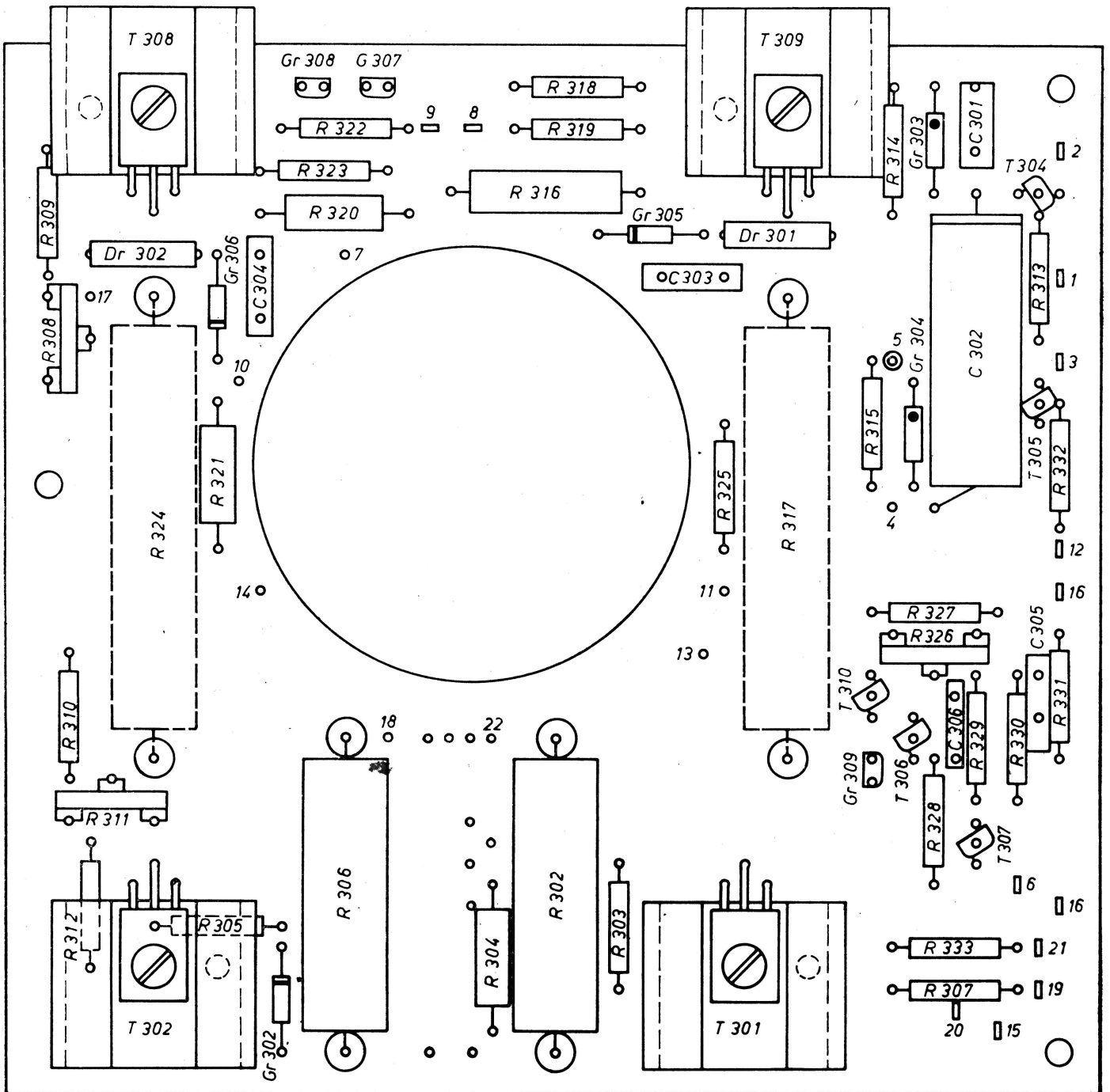
Leiterplatte Endstufe
