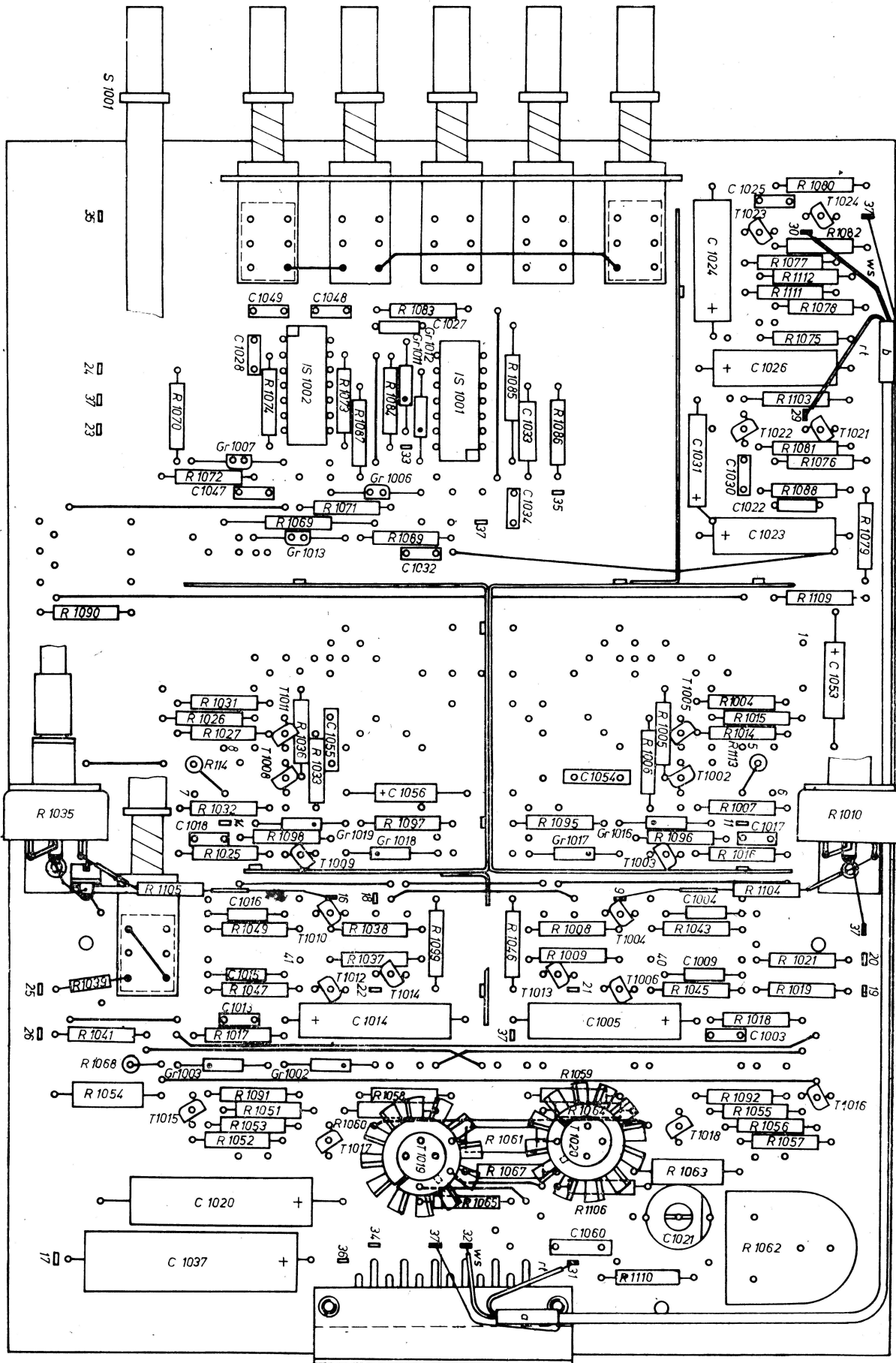
Leiterplatte Y-Kassette
